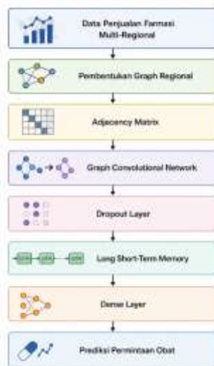
Gambar 2. Arsitektur GCN-LSTM
