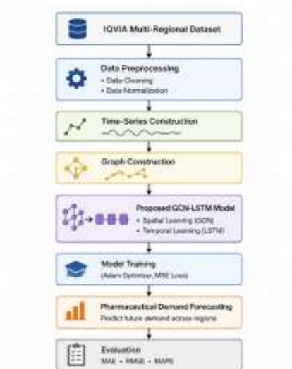
Gambar 1. Metodologi penelitian
