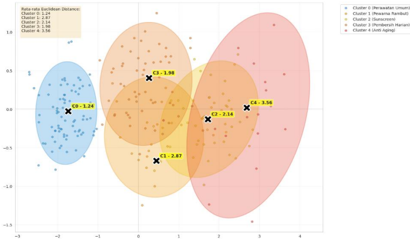
Gambar 3. PCA Clustering
